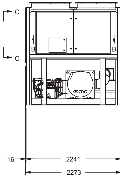
VIEW A-A
