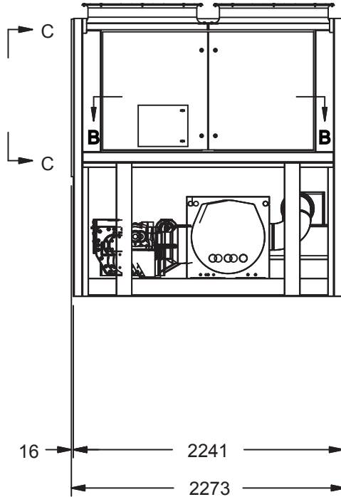
VIEW A-A
